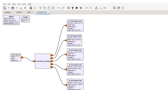
Figura 5: Diagrama de bloques del analizador estadístico de señales
