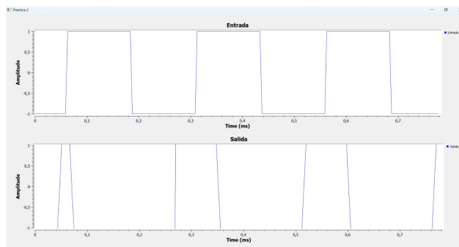
Figura 2: Simulación del funcionamiento del bloque acumulador.
